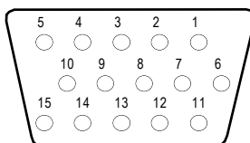
Connecteur VGA / SVGA (face arrière du modèle 85B)
