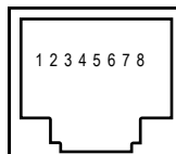
Schéma des connecteurs AUX1 et AUX2 (face arrière du modèle 85B)
