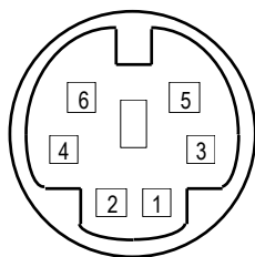
Connecteur clavier (face arrière du modèle 85B)
