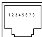
Schéma du connecteur LAN (face arrière du modèle 85B)
