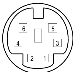
Connecteur souris (face arrière du modèle 85B)
