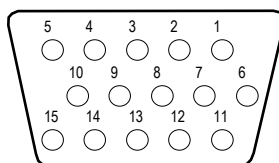
Connecteur VGA / SVGA (face arrière du modèle 75B)
