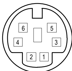
Connecteur souris (face arrière du modèle 75B)
