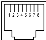
Schéma des connecteurs AUX1 et AUX2 (face arrière du modèle 75B)
