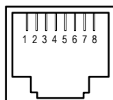
Schéma du connecteur LAN (face arrière du modèle 65B)
