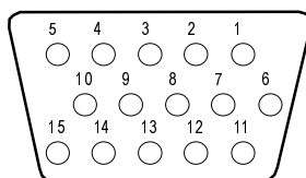
Connecteur VGA / SVGA (face arrière du modèle 56)
