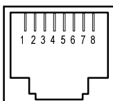
Schéma du connecteur AUX2 (face arrière du modèle 56)
