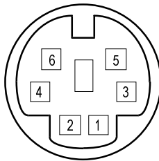
Connecteur clavier (face arrière du modèle 56)
